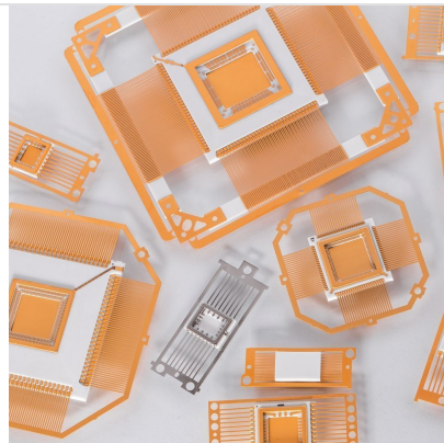
Корпус металлокерамический типа 4 4153.20-5
