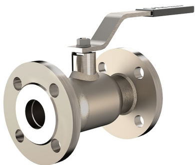
Кран шаровый 11лс72п Ду200 Ру 1,6-4,0МПа
