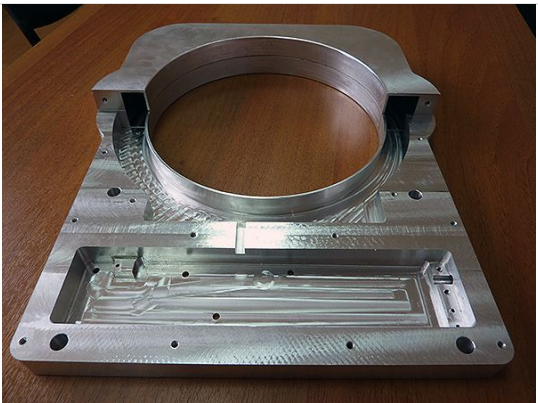
Алюминиевые корпуса для РЭА
