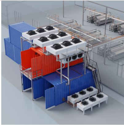
Скороморозильные комплексы на базе вертикально-плиточных аппаратов
