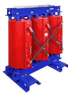
Сухой трансформатор с литой изоляцией серии Systeme3AL на номинальное напряжение 6-35 кВ и номинальную мощность до 10000 кВА
