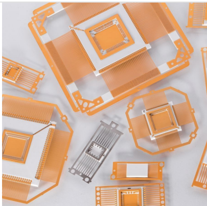
Корпус металлокерамический типа 4 4112.16-2.04
