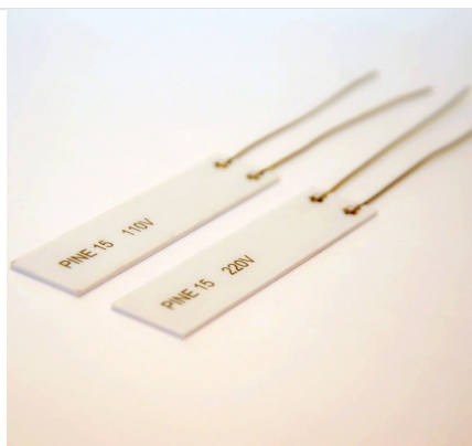
Плата металлокерамическая нагревательная ПМКН- 132-07 65*5*1ММ 380±80ОМ 220В
