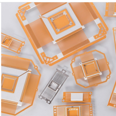
Корпус металлокерамический типа 4 4112.16-3.04 УФ0.487.005 ТУ АО «ЗПП» Россия
