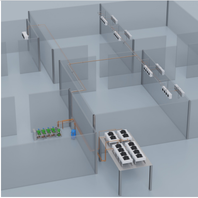
Промышленное холодильное оборудование для склада
