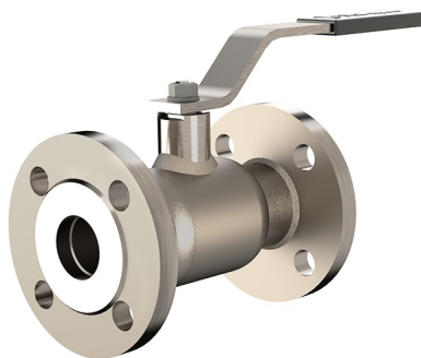
Кран шаровый 11нж72п Ду32 Ру 1,6-4,0МПа
