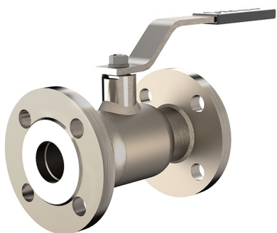
Кран шаровый 11лс72п Ду50 Ру 1,6-4,0МПа
